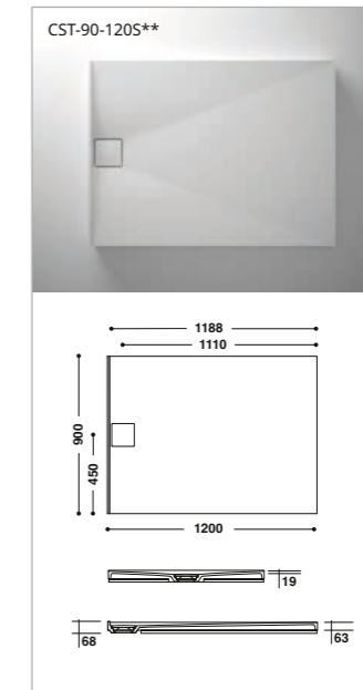
**Afvoer aan de zijkant
