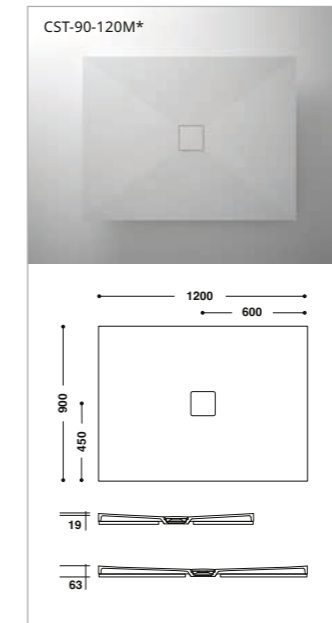
*Afvoer in het midden
